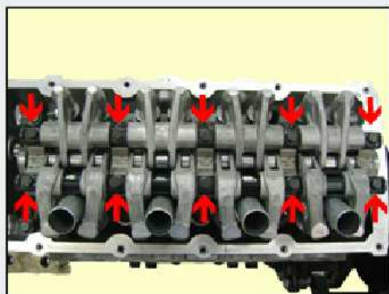
PARAFUSOS DE FIXAÇÃO DO GUIA DA CORRENTE 23,7 Nm [2,3 kgm]
