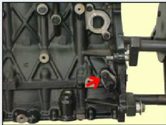
PARAFUSO DE FIXAÇÃO DO SENSOR DE DETONAÇÃO 21,3 Nm [2,1 Kgm]
