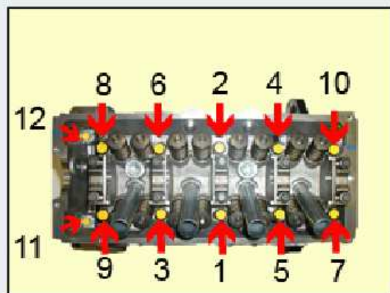
PARAFUSOS DE FIXAÇÃO DOS EIXOS / BALANCINS 27,1 Nm [2,7 kgm]
